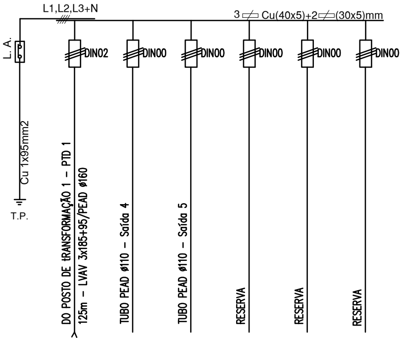
ARMÁRIO DE DISTRIBUIÇÃO 2 - AD 2 Tipo W (2T2+4T00)
