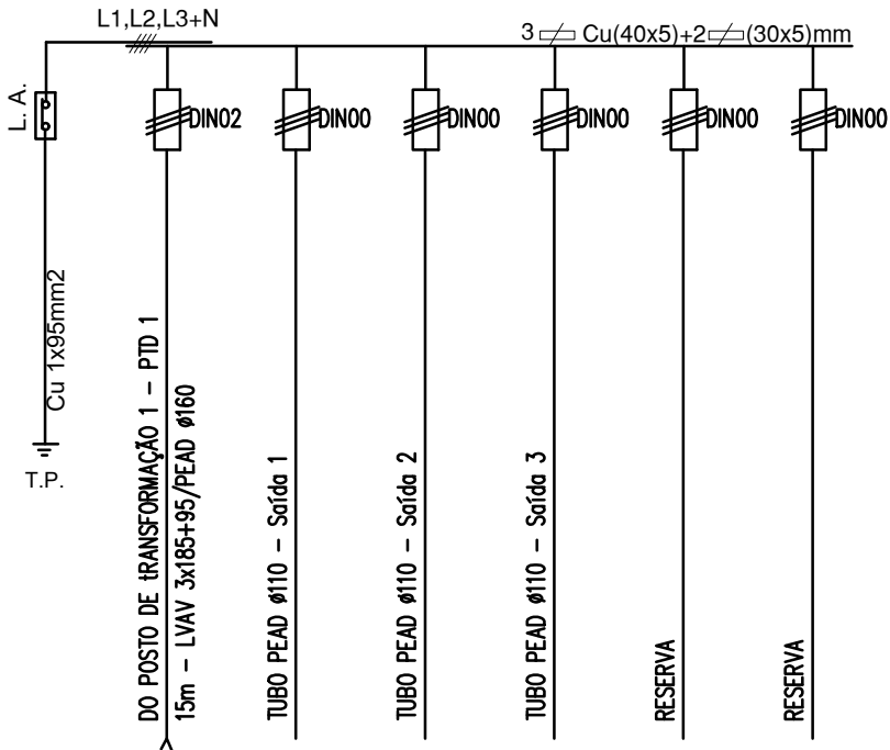
ARMÁRIO DE DISTRIBUIÇÃO 1 - AD 1 Tipo W (2T2+4T00)
