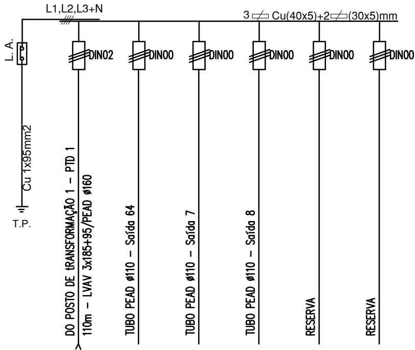
ARMÁRIO DE DISTRIBUIÇÃO 3 - AD 3 Tipo W (2T2+4T00)
