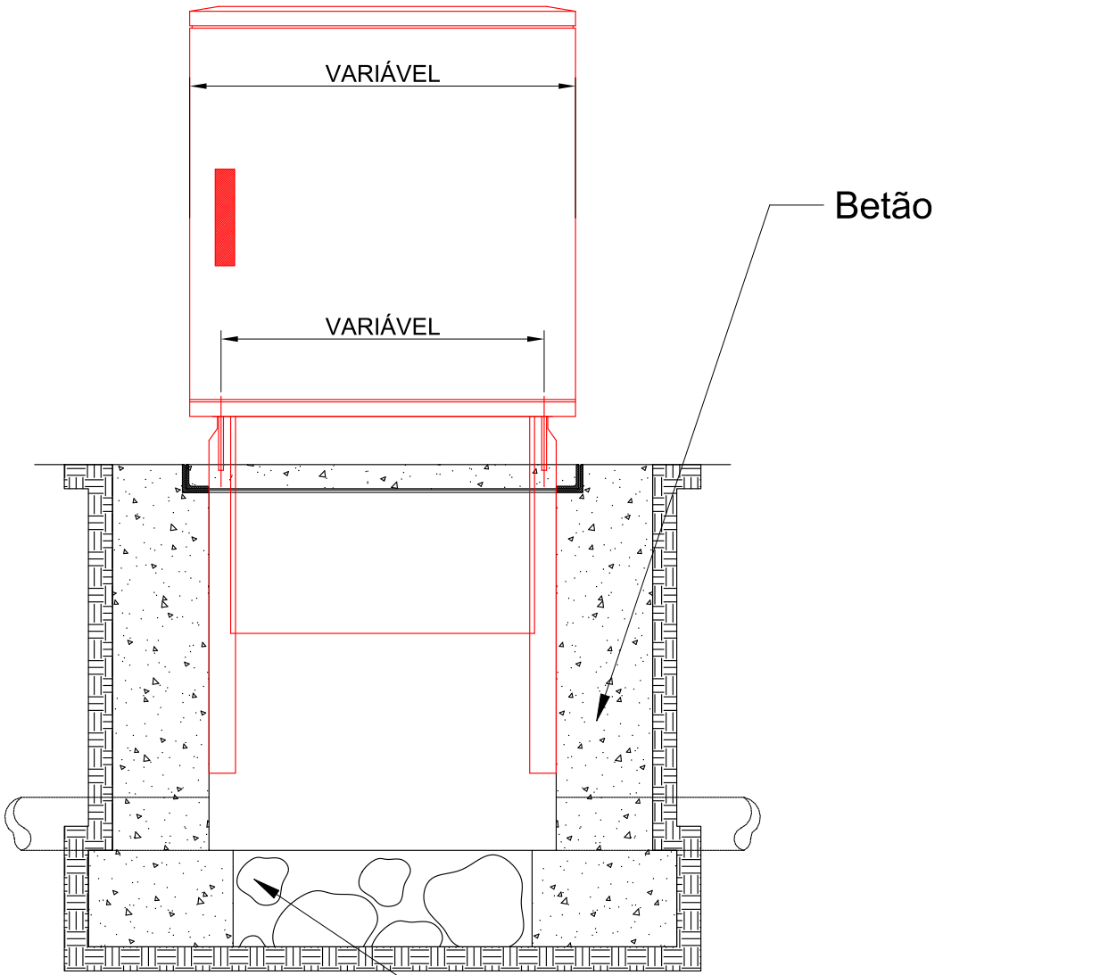
CORTE C-D
