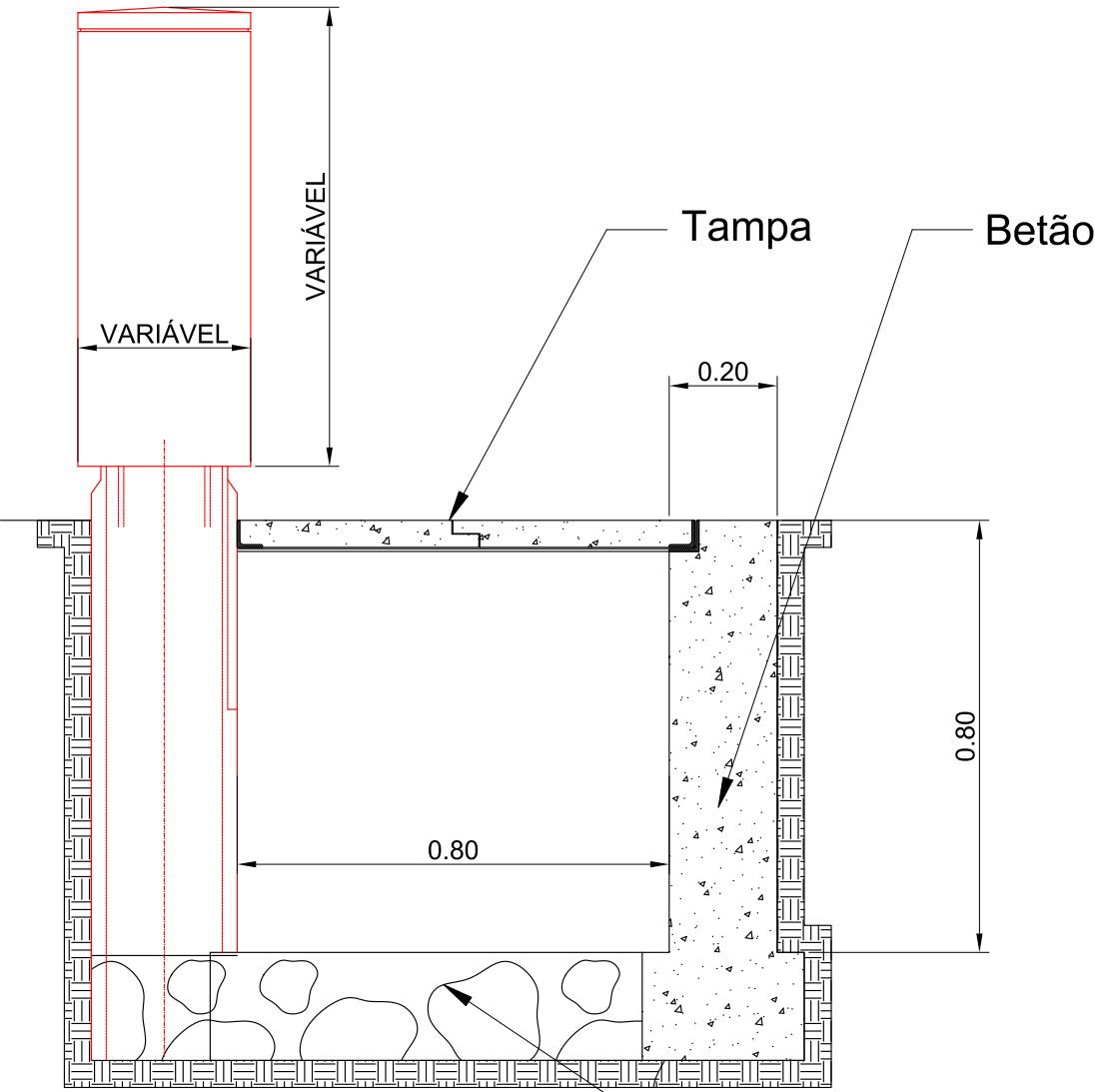
CORTE A-B
