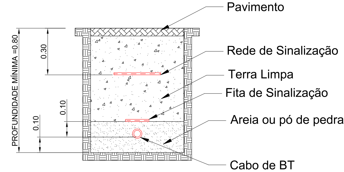
COLOCAÇÃO DE CABOS DE BAIXA TENSÃO DIRECTOS EM VALA CORTE TIPO
